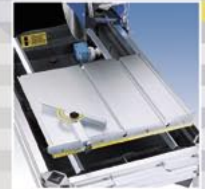
De aluminium zaagwagen loopt met 6 gelagerde wielen over de roestvrijstalen rails: uiterste precisie en duurzaamheid
